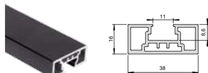
Perfil vertical
