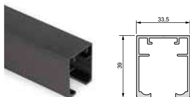
Guía Flat
