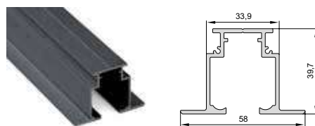
Guía Ras
