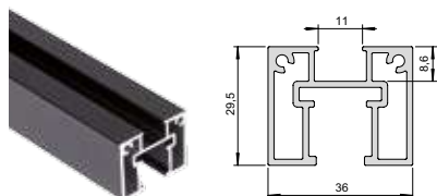
Perfil horizontal
