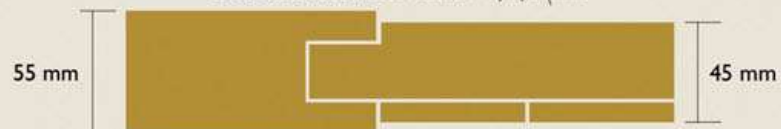
Sección Puerta / Door section / قسم الباب
